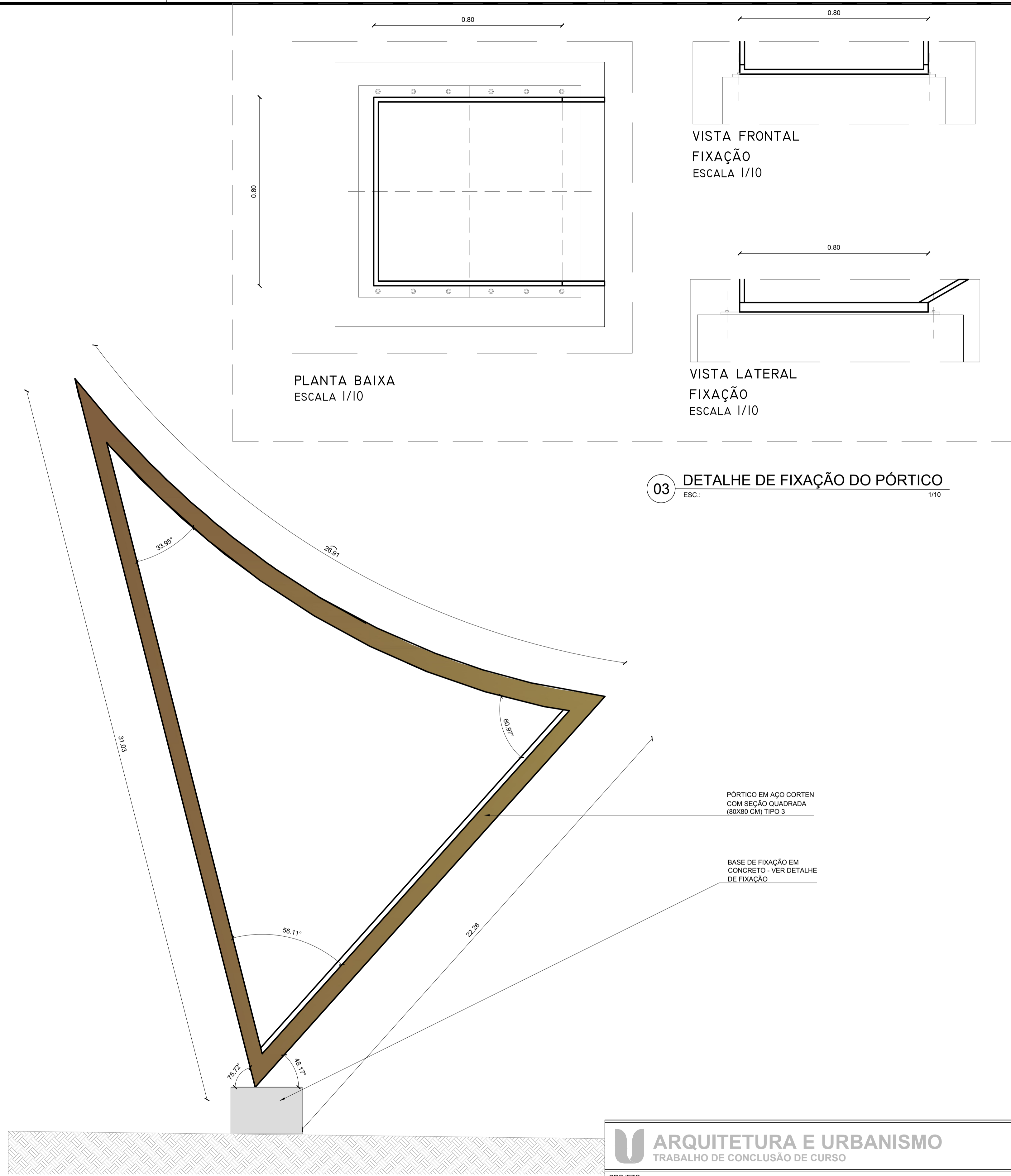
02 ESTRUTURA METÁLICA - VISTA DO PÓRTICO TIPO 3 ESC.: 1/100
