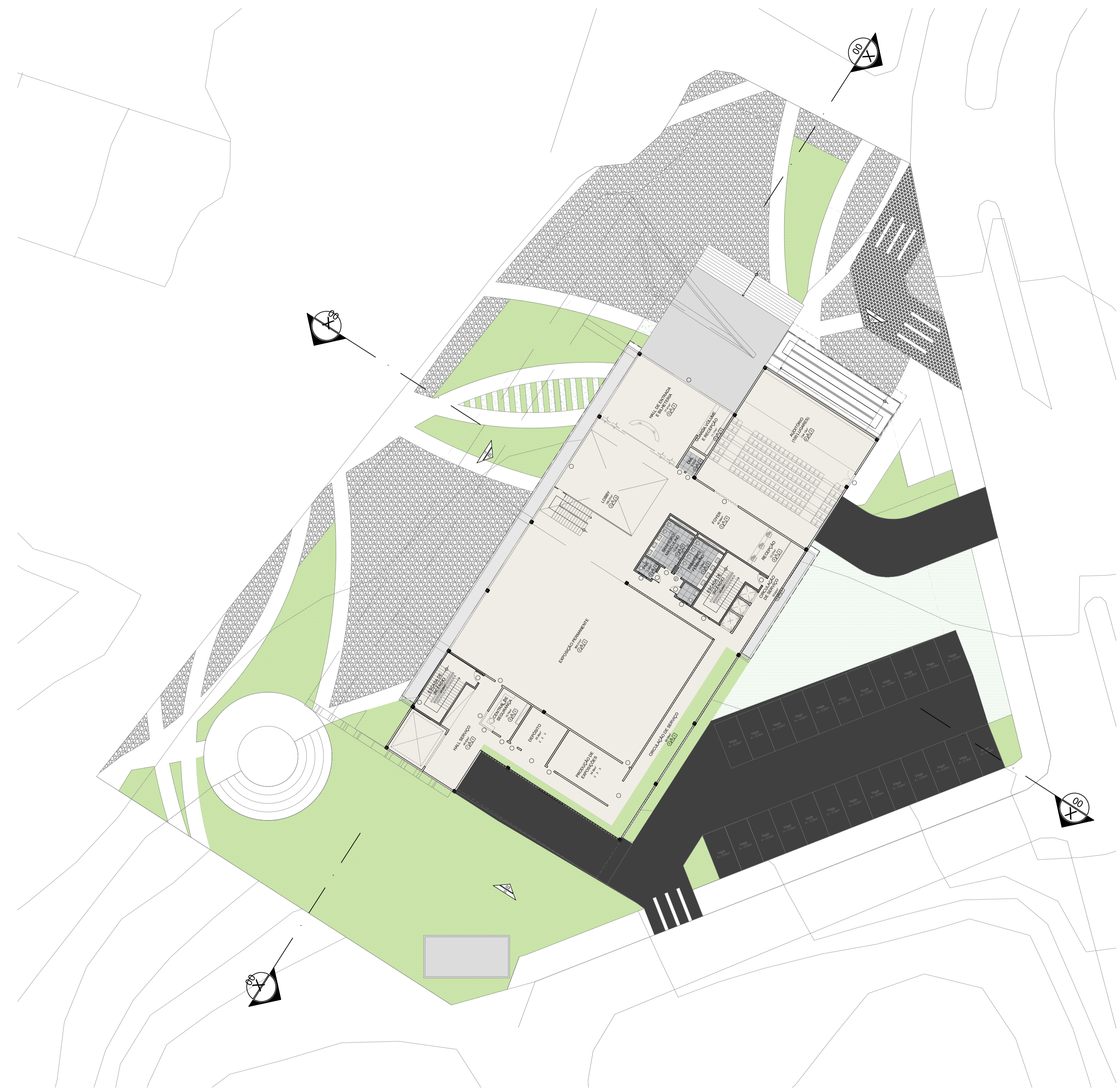
01 PLANTA BAIXA GERAL TÉRREO - ACESSO PRINCIPAL ESC.: 1/250
