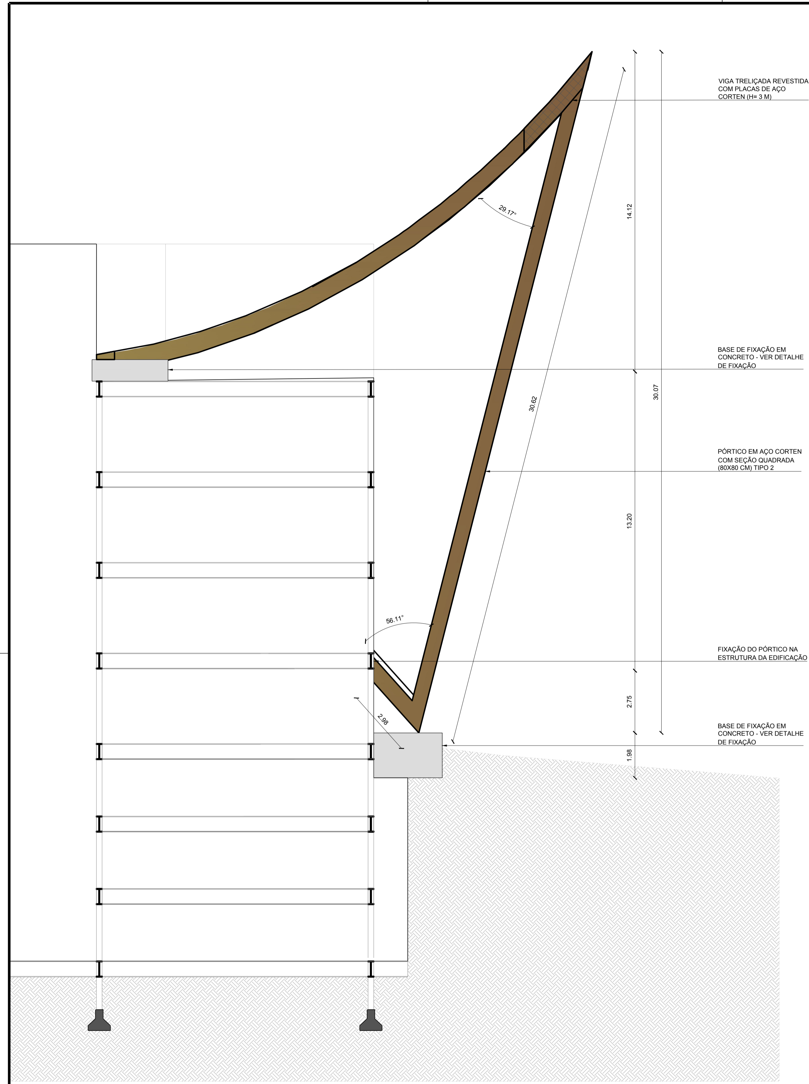
01 ESTRUTURA METÁLICA - CORTE DO PÓRTICO TIPO 2 ESC.: 1/100
