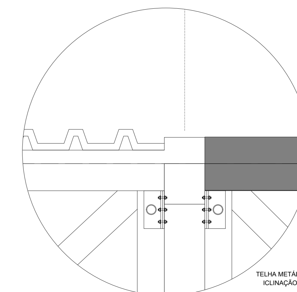
10 DETALHE ESC.: 1/20
