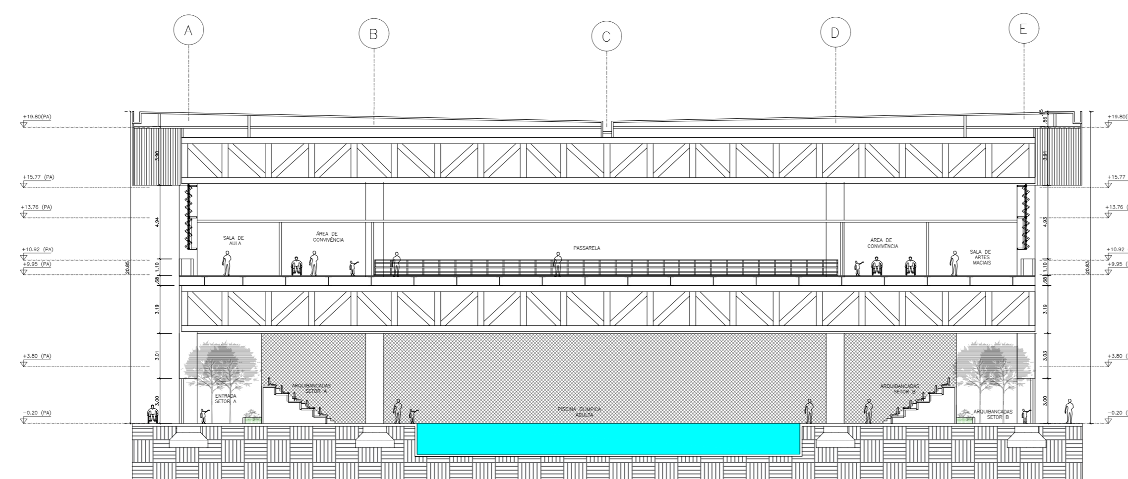
08 CORTE EE ESC.: 1/250
