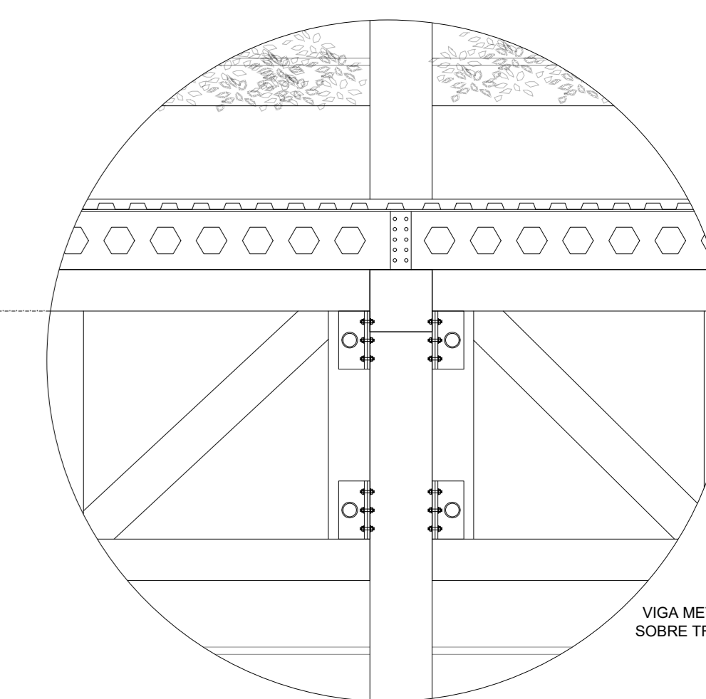
09 DETALHE ESC.: 1/20
