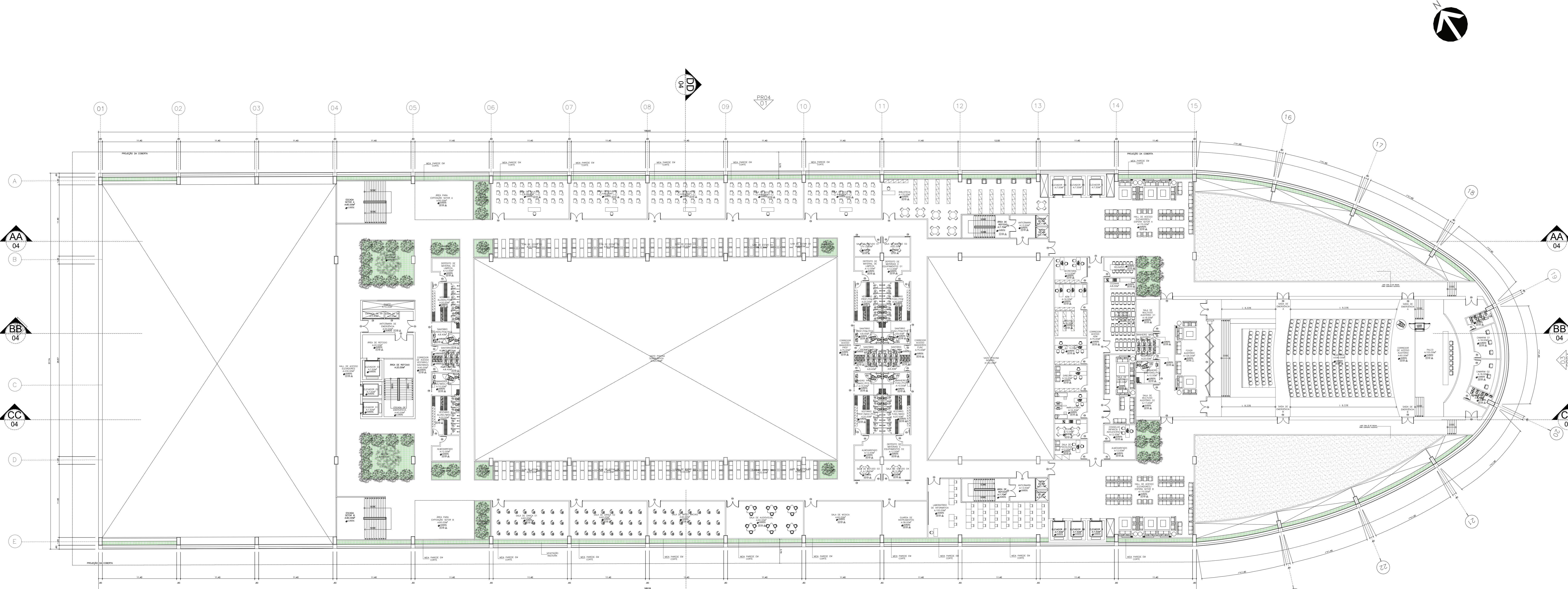
04 PLANTA PRIMEIRO PAV ESC. 1/250
