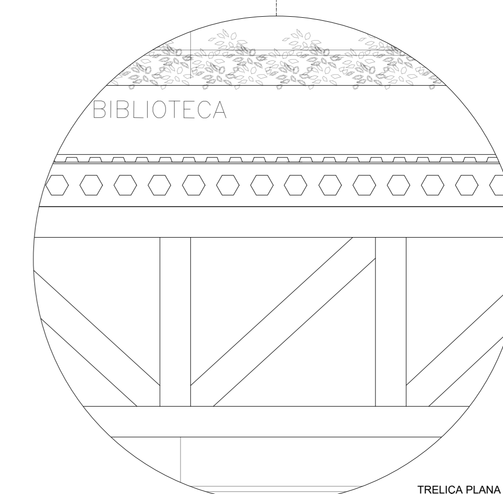
12 DETALHE ESC.: 1/20
