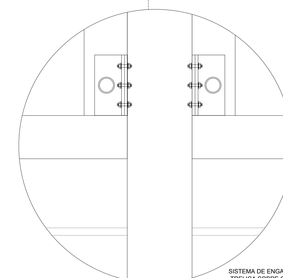
11 DETALHE ESC.: 1/20
