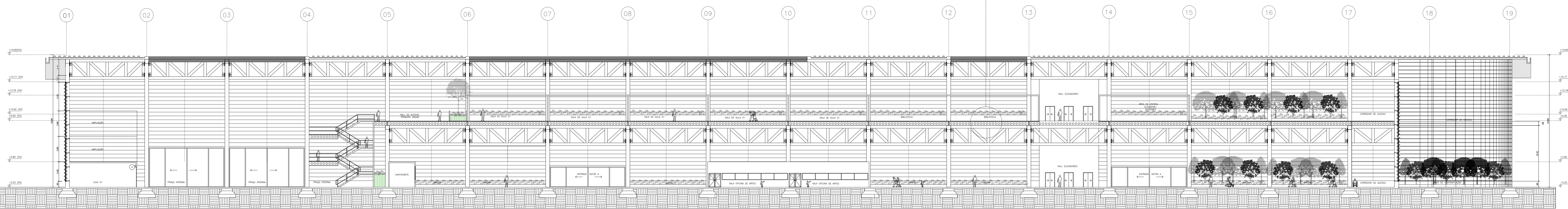
05 CORTE AA ESC.: 1/250
