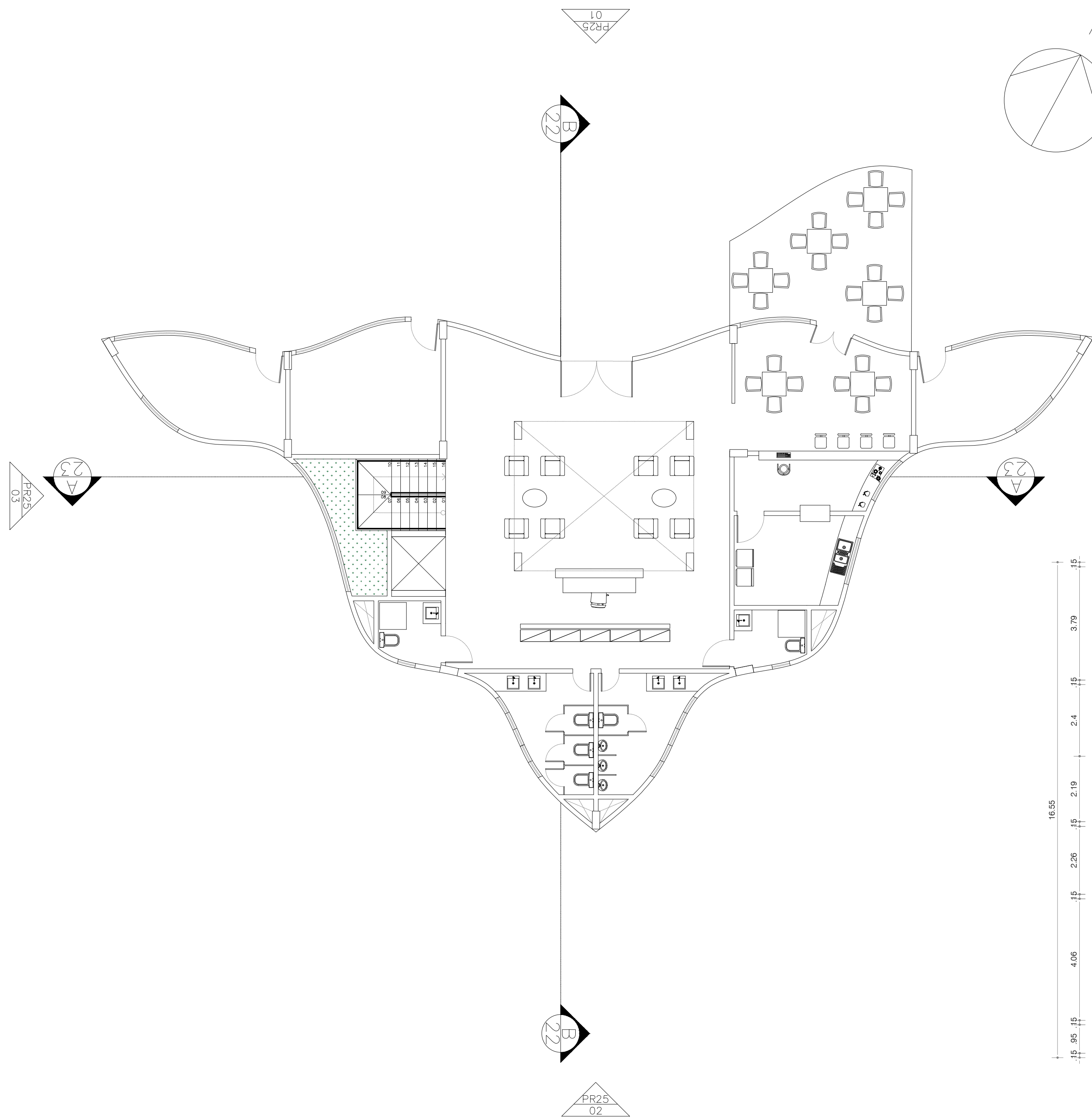
18 PLANTA BAIXA - TÉRREO (LAYOUT) - COWORKING ESC.: 1/100
