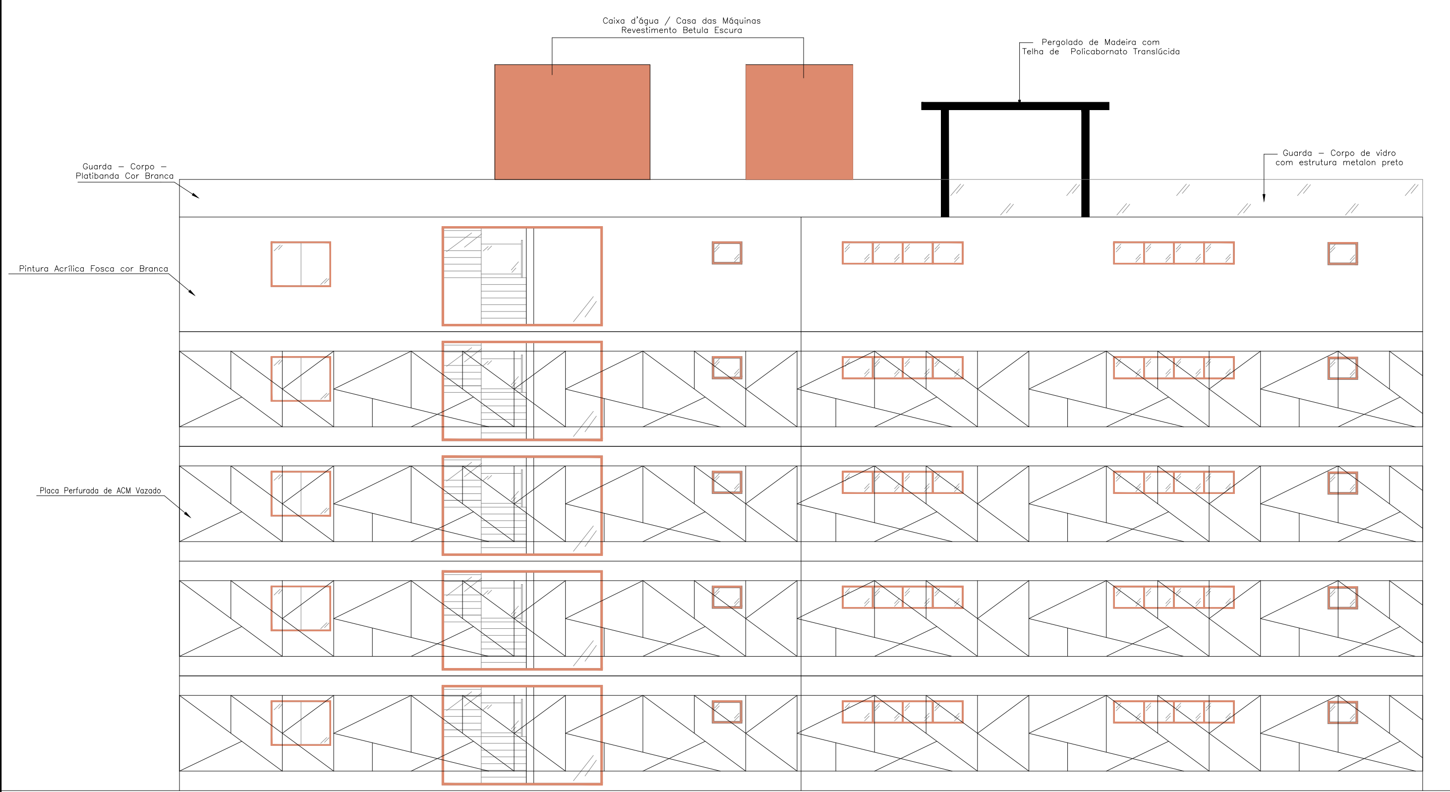
36 FACHADA 01 - COWORKING ESC.: 1/100
