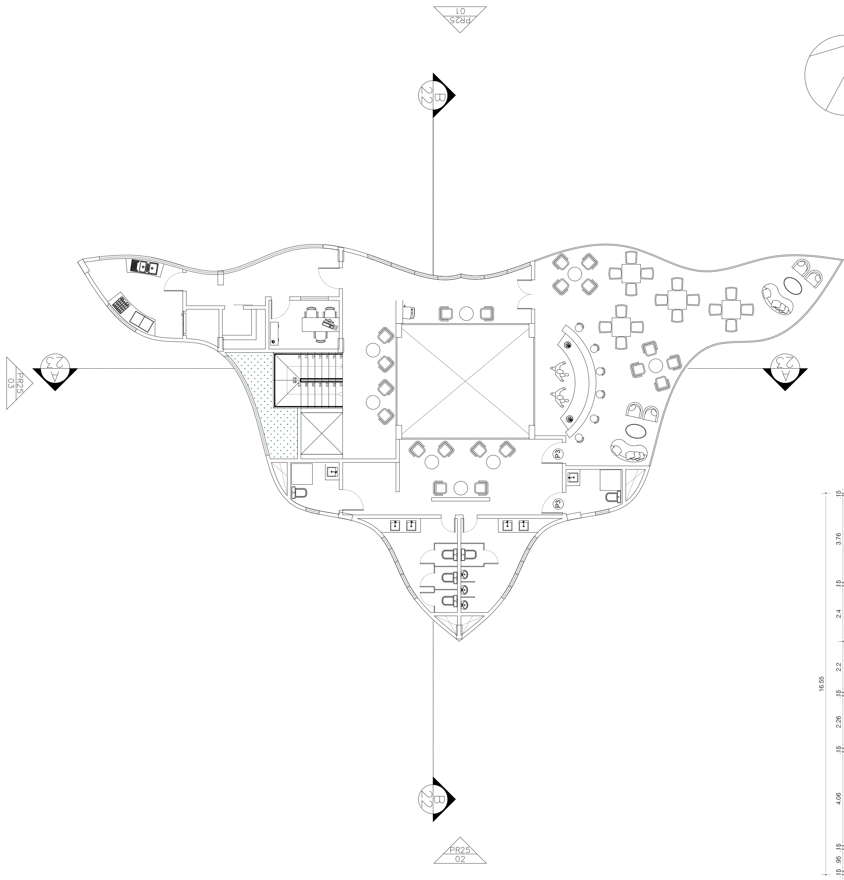
26 PLANTA BAIXA - 4º PAV. (LAYOUT) - COWORKING ESC.: 1/100
