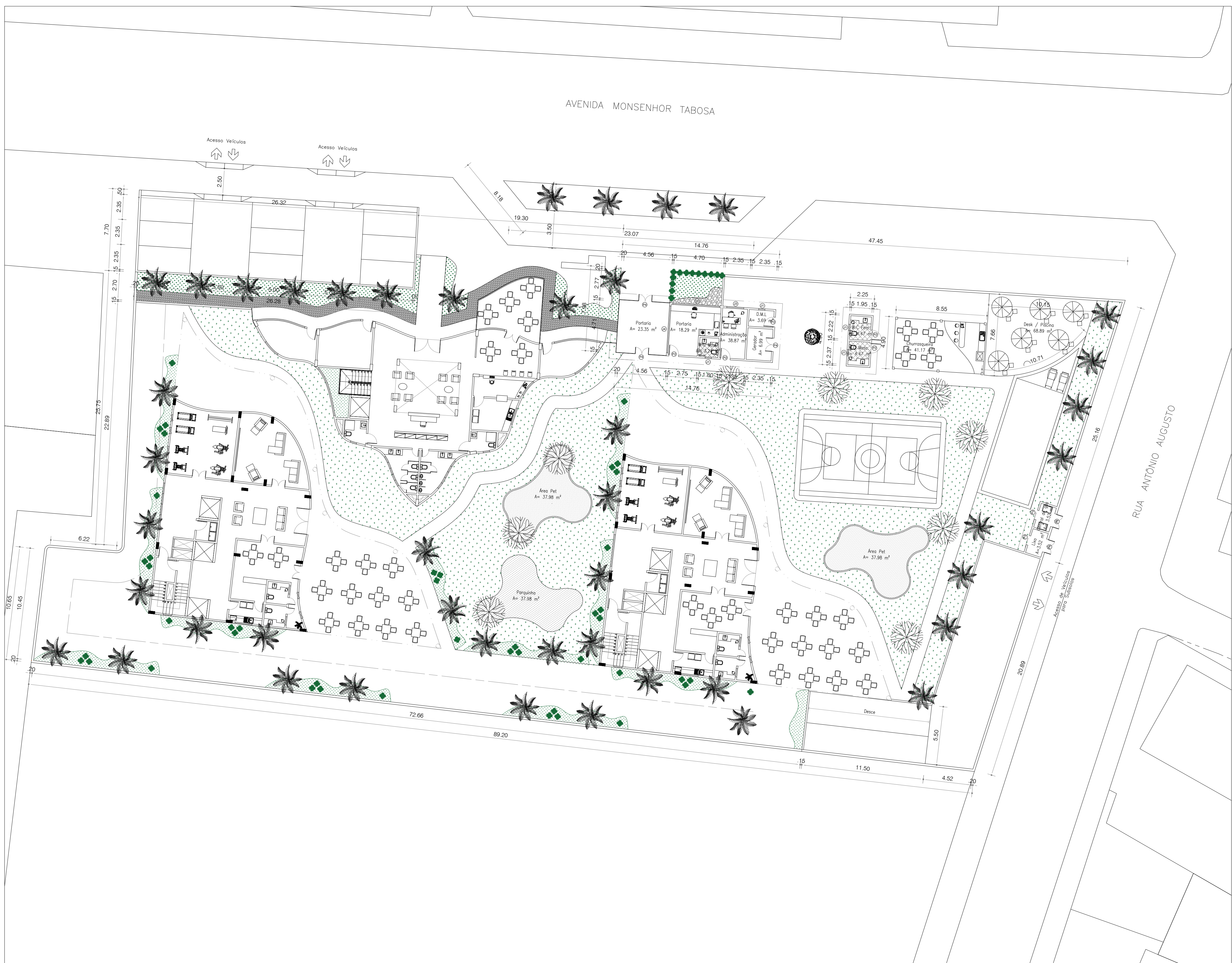
03 PLANTA BAIXA - GERAL ESC.: 1/200
