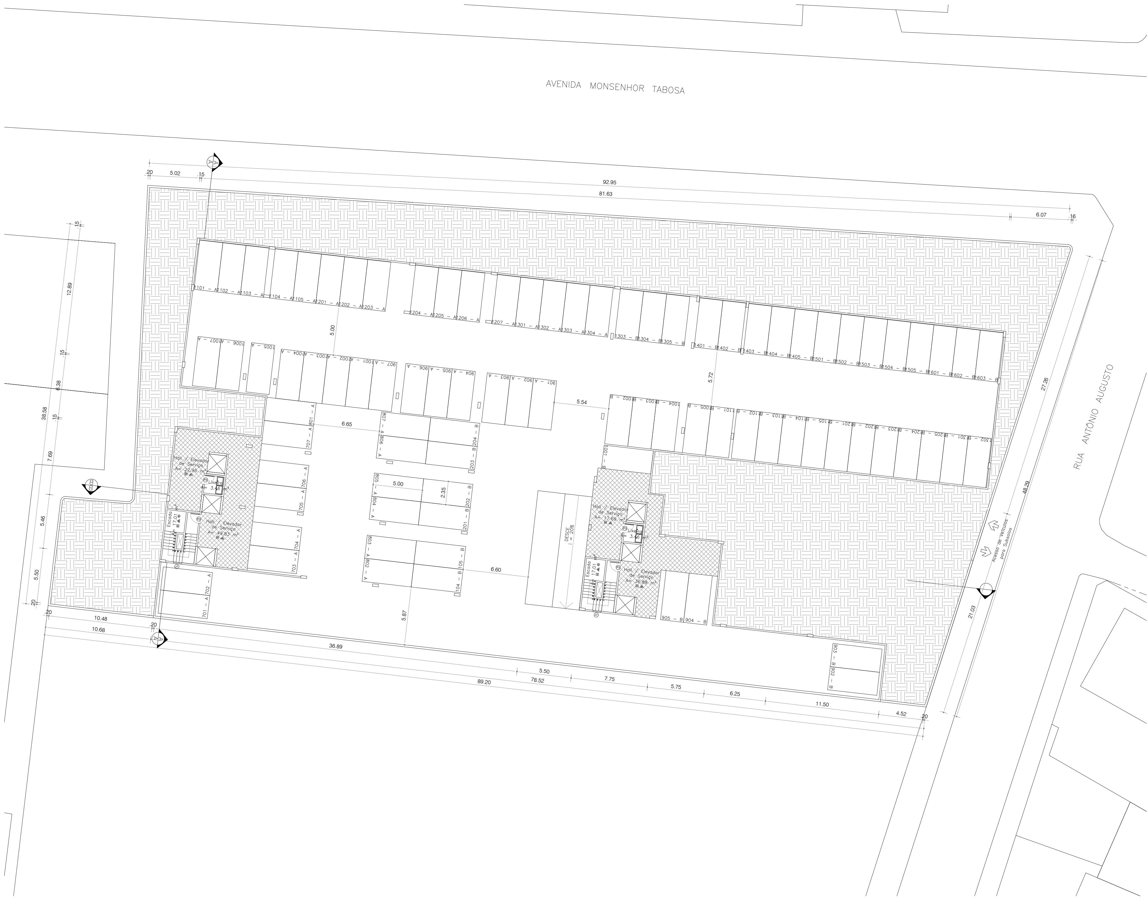
06 PLANTA BAIXA - SUBSOLO 02 ESC.: 1/200
