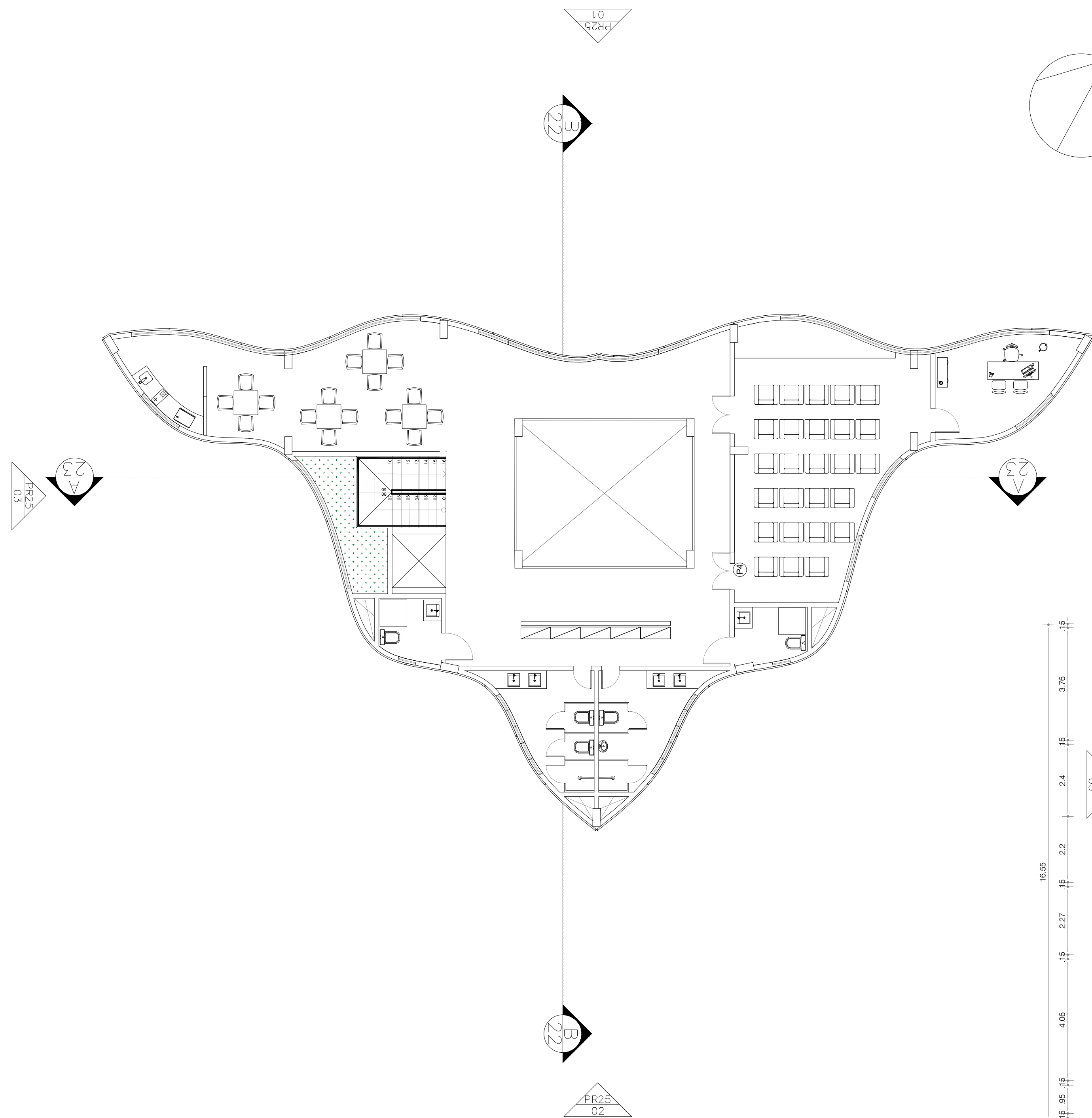
24 PLANTA BAIXA - 3º PAV. (LAYOUT) - COWORKING ESC.: 1/100
